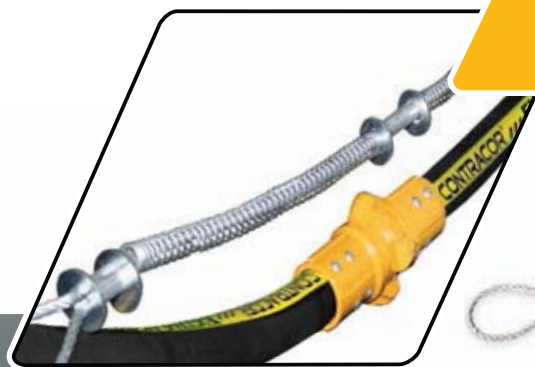
Гальванизированный стальной тросик с подпружиненными алюминиевыми муфтами
