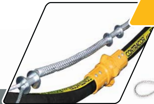
Гальванизированный стальной тросик с подпружиненными алюминиевыми муфтами
